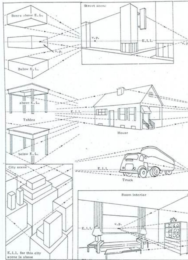
ภาพร่างเส้นทัศนียภาพแบบจุดรวมสายตาสองจุด
